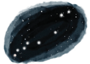
Rys
