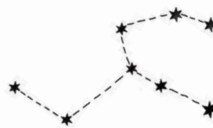
Žirafa
