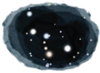
Kasiopeja
