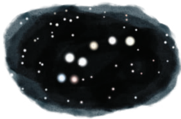
Malý medvěd
