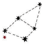
Ceteus
