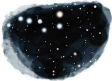
Velká medvědice
