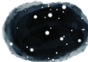
Žirafa
