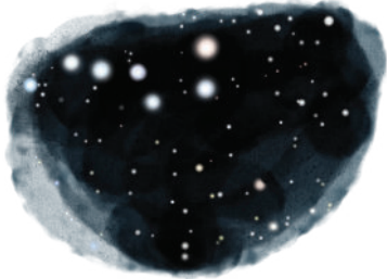
Velká medvědice
