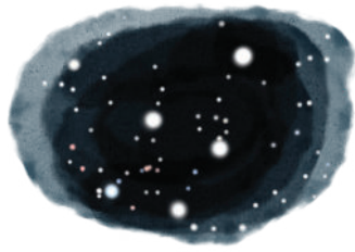
Ceteus
